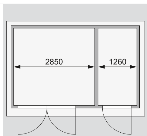
Draufsicht / Innenmaße
