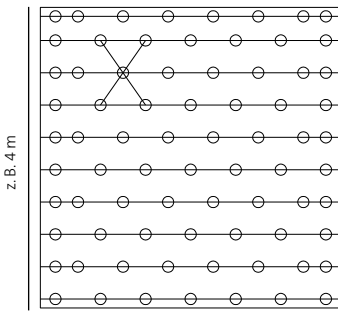
Unterkonstruktion
