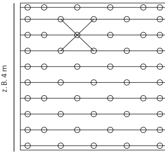
ALU-Unterkonstruktion
