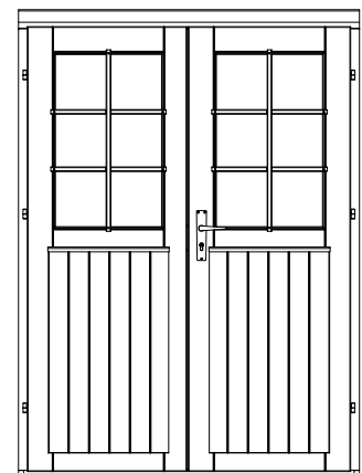
Nr. 13 Double door 1425 x 1955 mm 40 mm
