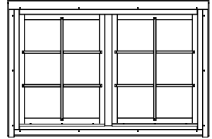
Nr. 14-2 Window 40 mm 1530 x 990 mm
