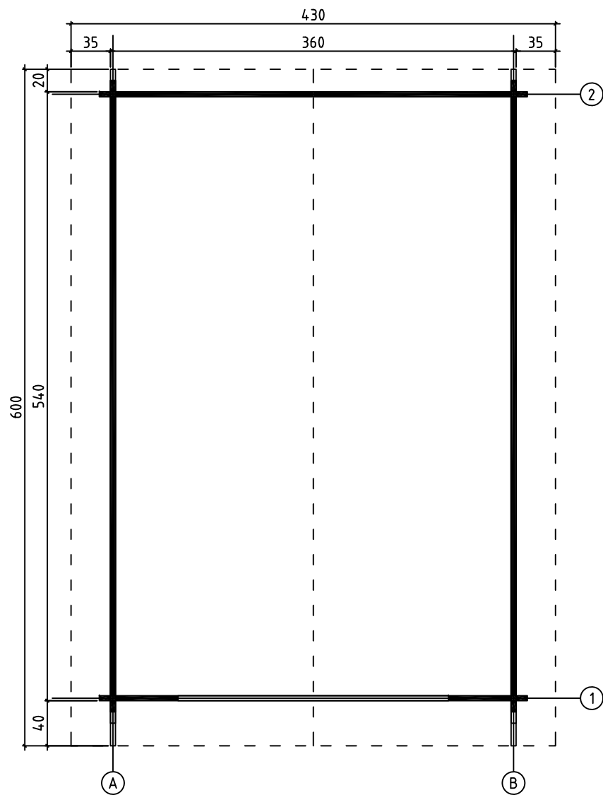
GROUNDPLAN - GRUNDPLAN - PLAN DE MASSE
